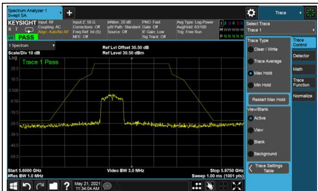
802.11ac (VHT40) - 5755MHz
