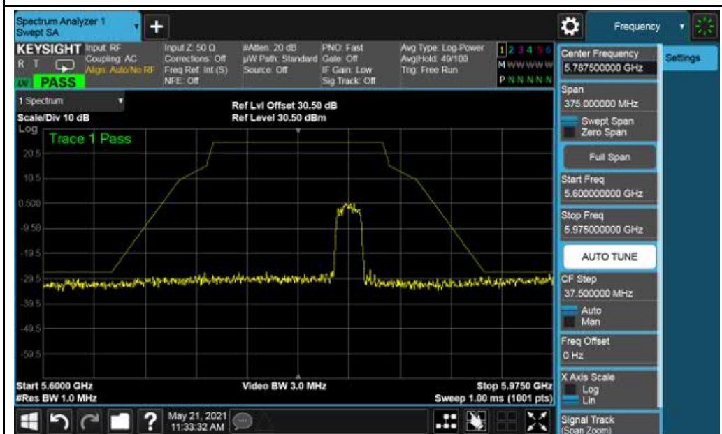
802.11ac (VHT20) – 5825MHz
