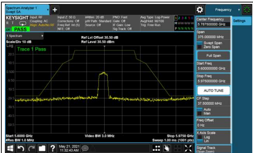
802.11ac (VHT20) – 5785MHz
