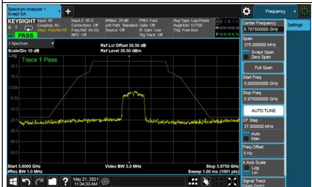
802.11ac (VHT40) - 5795MHz
