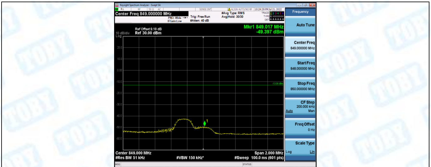
Band5-3MHz-QPSK-20635-1RB#14
