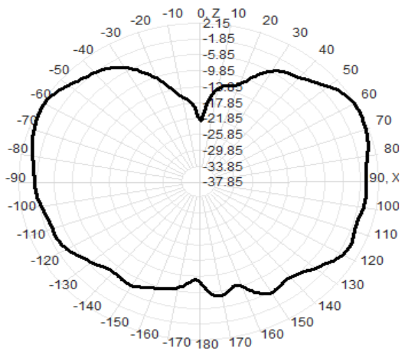
E(460MHz)
