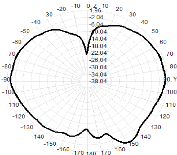
E(450MHz)
