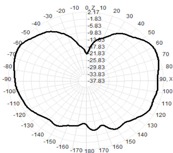
E(470MHz)
