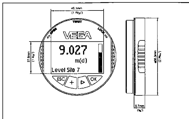
Fig. 28: PLICSCOM
