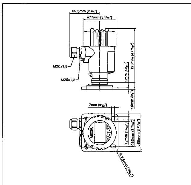
Fig. 27: VEGADIS 61
