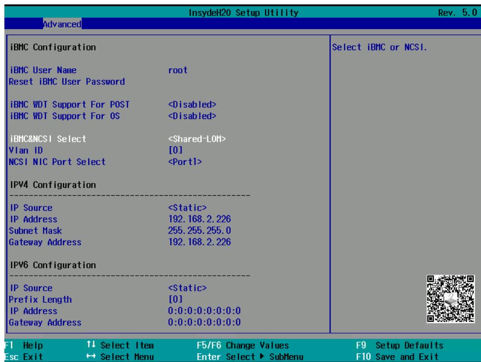
图 4-13 “BMC Configuration” 界面
