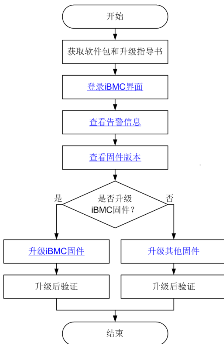
图 3-33 升级固件的流程
