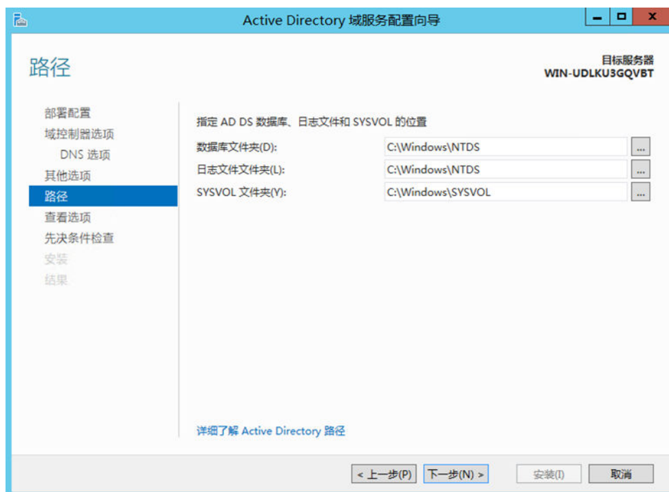
图 6-12 域服务路径
