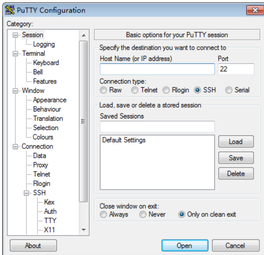
图 6-2 PuTTY Configuration
