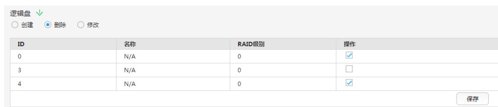
图 3-13 删除逻辑盘
