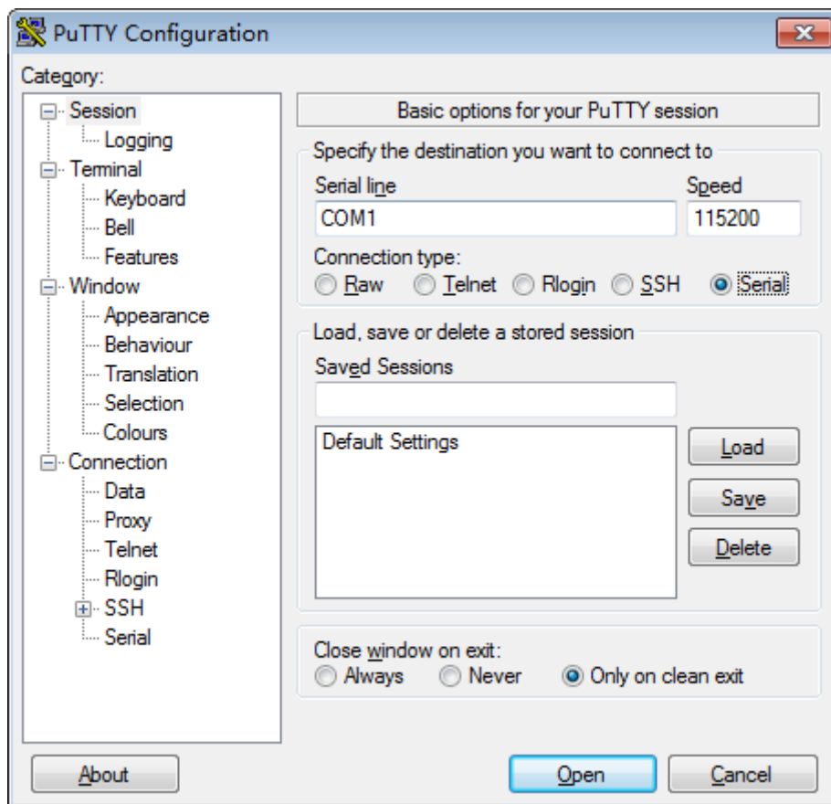
图 6-1 PuTTY Configuration
