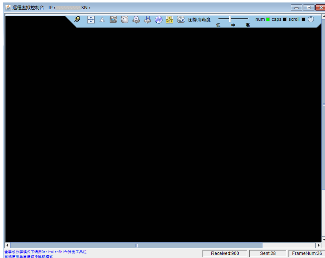
图 3-35 KVM 窗口
