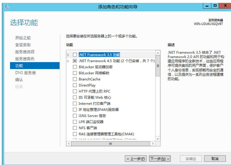
图 6-7 选择功能
