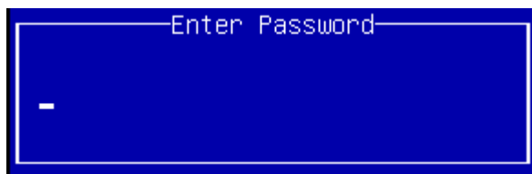
图 4-7 输入密码
