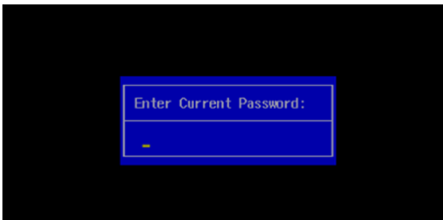
图 4-12 输入密码
