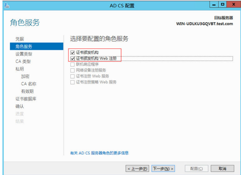
图 6-15 角色服务
