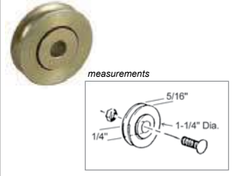
4-114 Sliding Glass Door Roller
