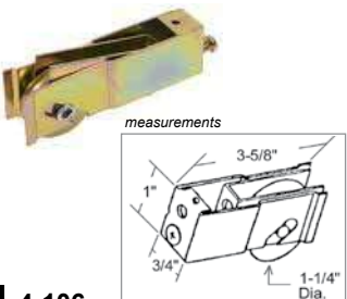
4-106 Sliding Glass Door Roller
