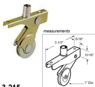
3-215 Sliding Screen Door Roller
