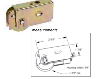
4-111 Sliding Glass Door Roller
