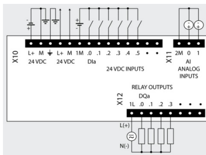
6ES7 211-1HE40-0XB0
