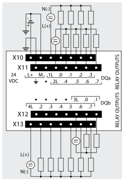
6ES7 222-1HH32-0XB0
