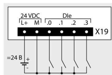
6ES7 221-3BD30-0XB0
