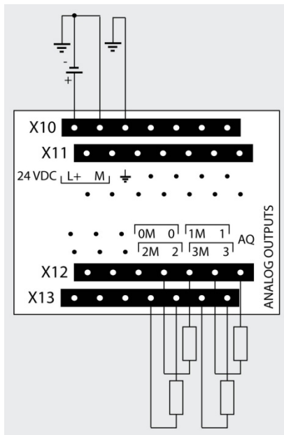
6ES7 232-4HD32-0XB0
