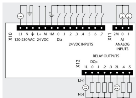
6ES7 212-1BE40-0XB0
