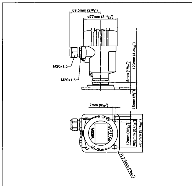
Fig. 27: VEGADIS 61
