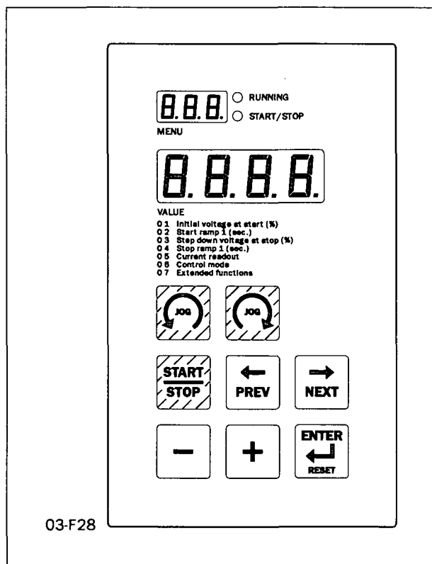
Fig. 13 PPU unit.
